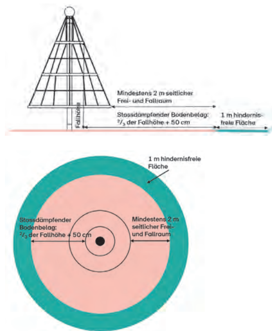
Abbildung 25 Hindernisfreie Fläche bei drehbaren Klettertürmen
