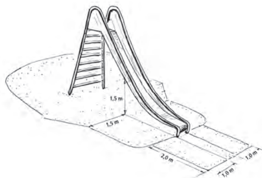
Abbildung 21 Aufprallfläche Rutsche
